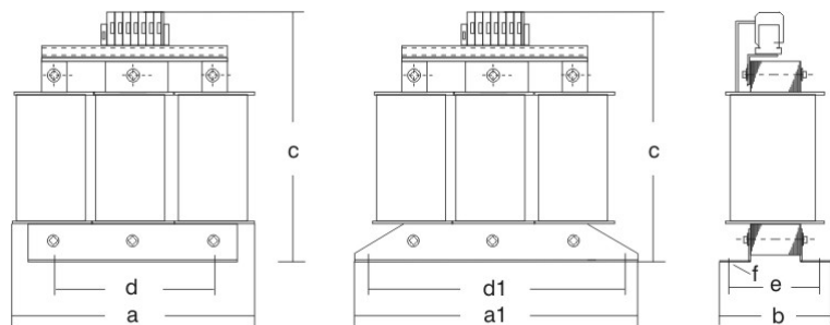
Standardausführung Bef.-Maße nach DIN 41307
